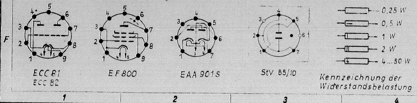
Sockelschaltbilder von unten gesehen
