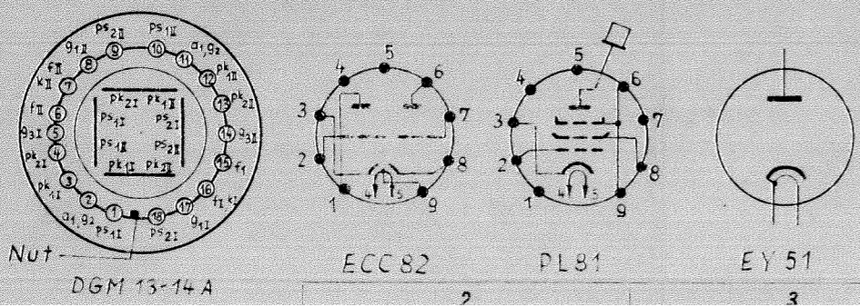
Sockelschaltbilder von unten gesehen
