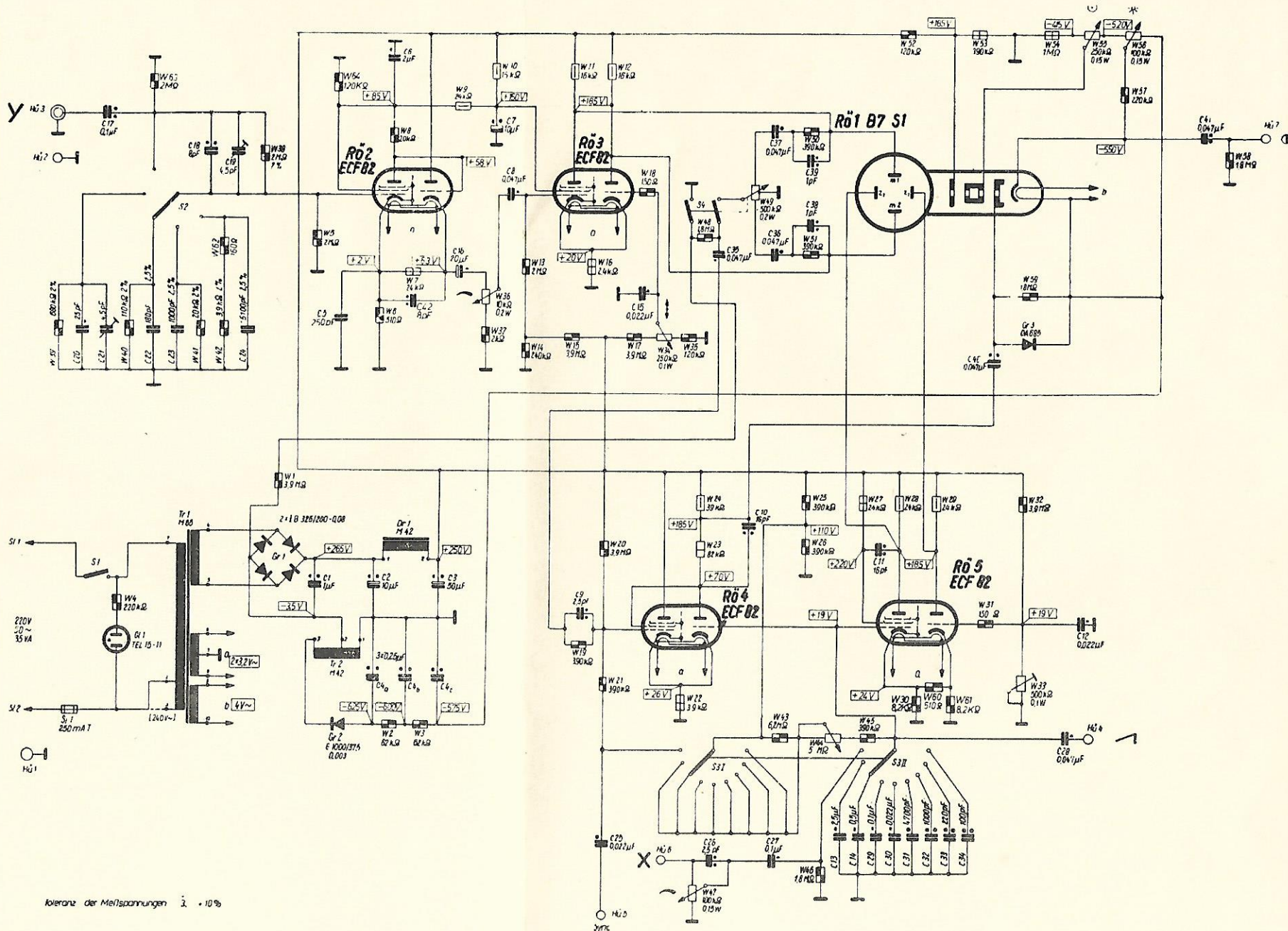
Wirkschaltnplan EO 1/7
